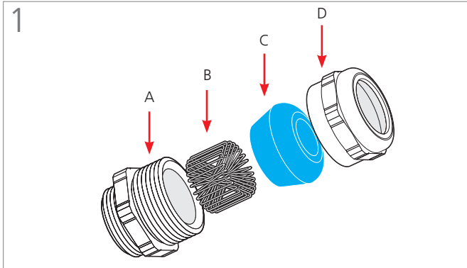
Bestandteile: Doppelnippel (A), Feder (B), Globe-Dichteinsatz (C), Druckschraube (D)
