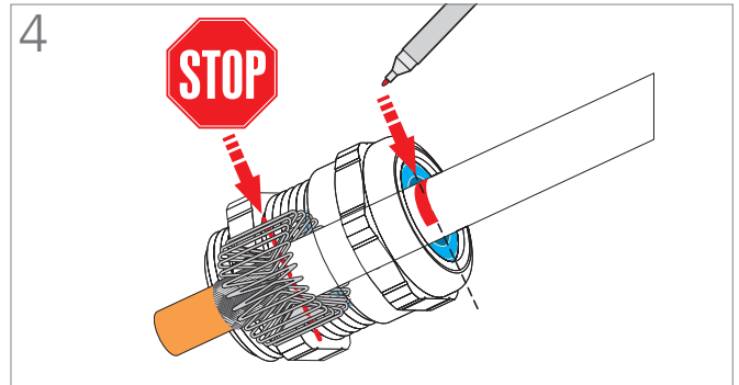
Markieren, wenn der Kabelmantel die Feder berührt
