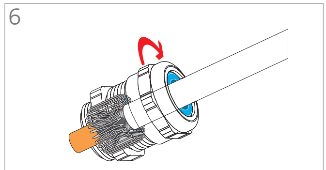
Druckschraube mit Anzugsdrehmoment festziehen (siehe Tabelle unten)
