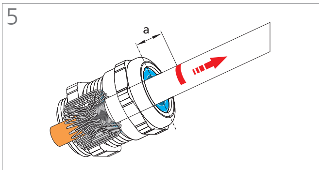
Kabel gemäß Maß a zurückziehen (siehe Tabelle unten)
